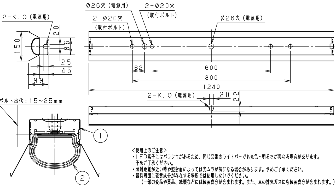
断面詳細図
