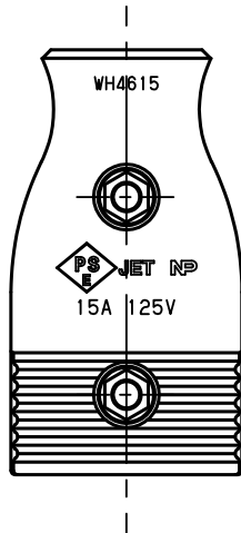
裏面刻印図
