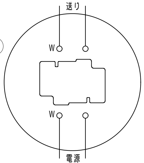
結線図（裏面図）
