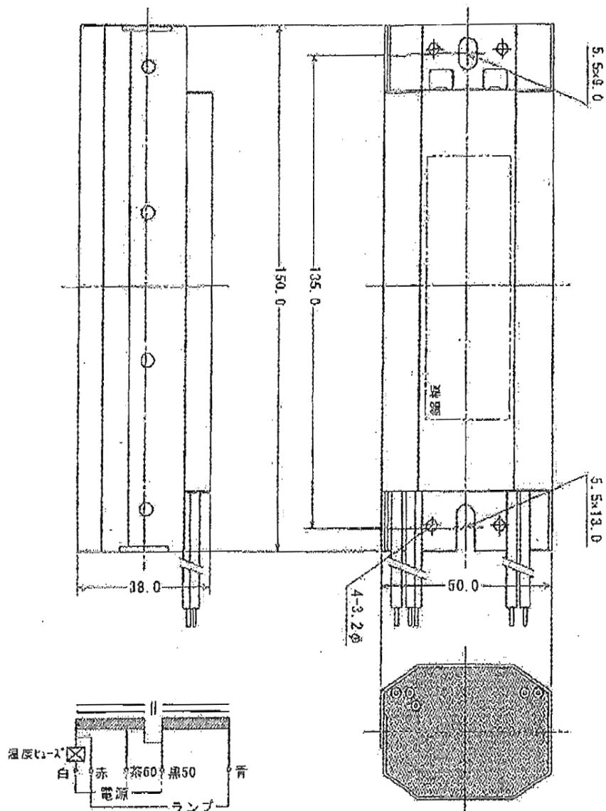
配線図
