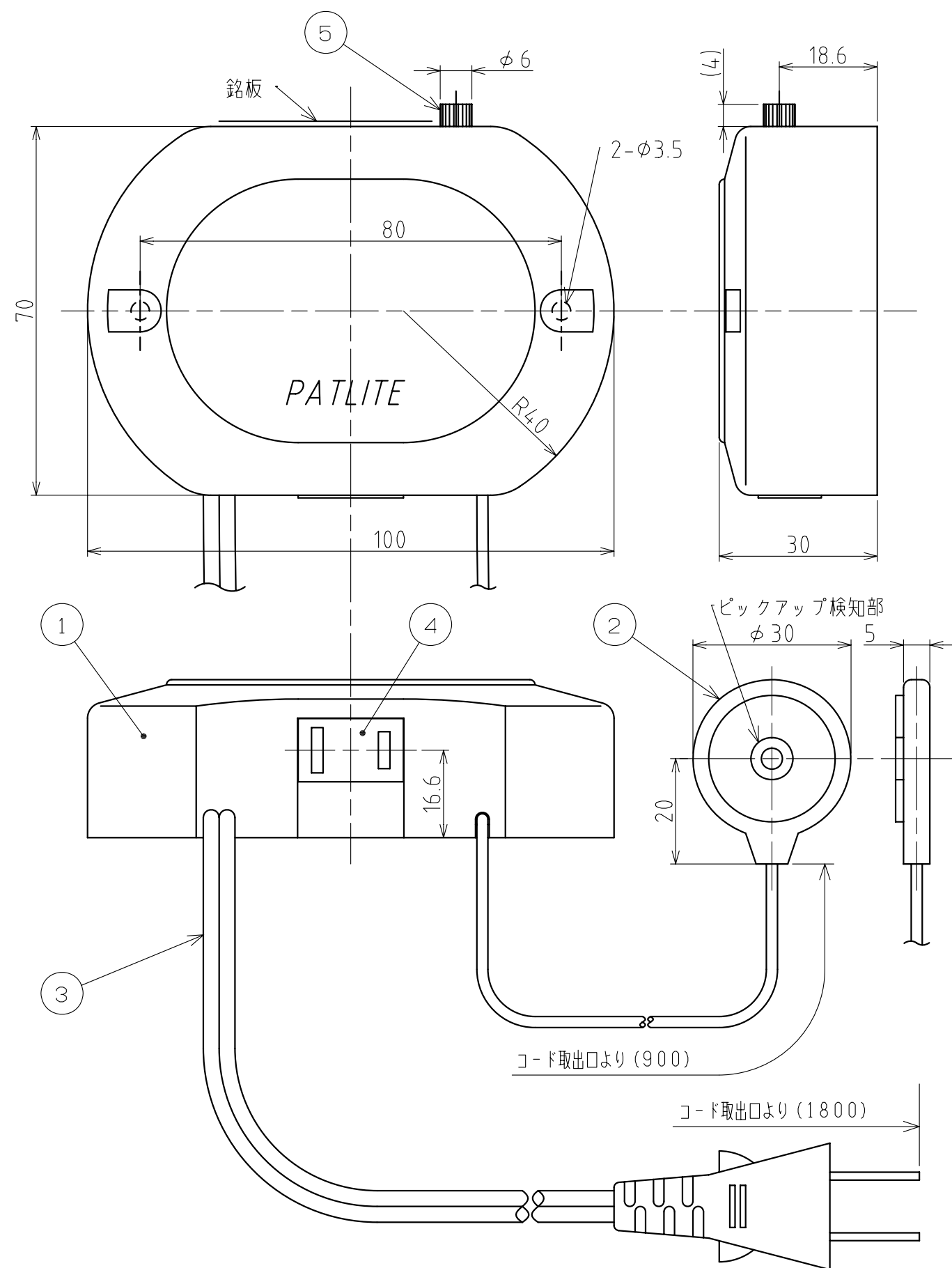
外観寸法図
