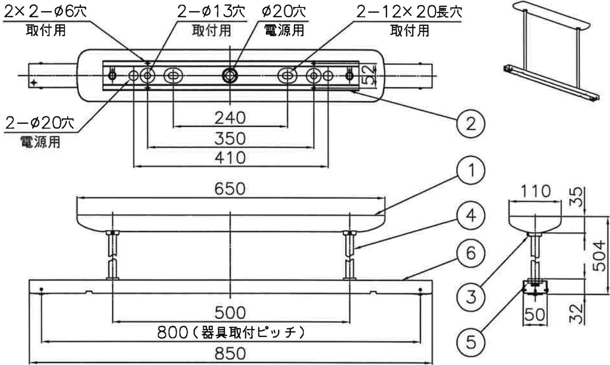
断面詳細図1/3
