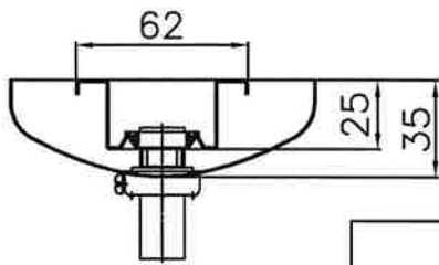
断面詳細図1/3
